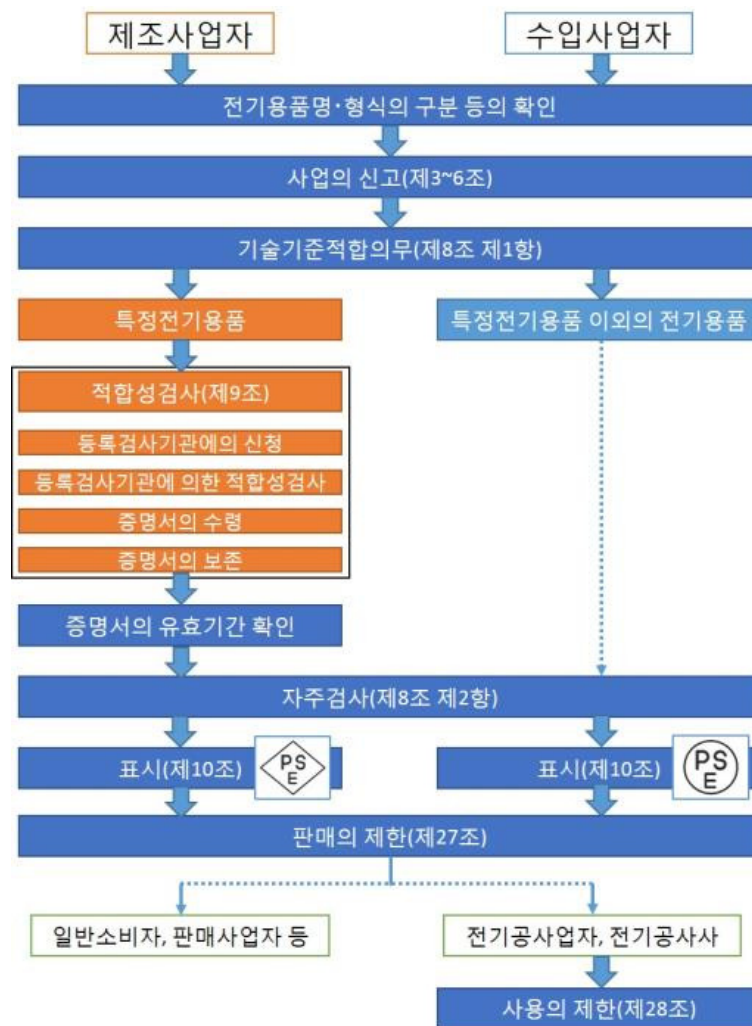
〈그림 3-13〉 전기용품안전법의 업무 절차 흐름도(제품 유통 전)
