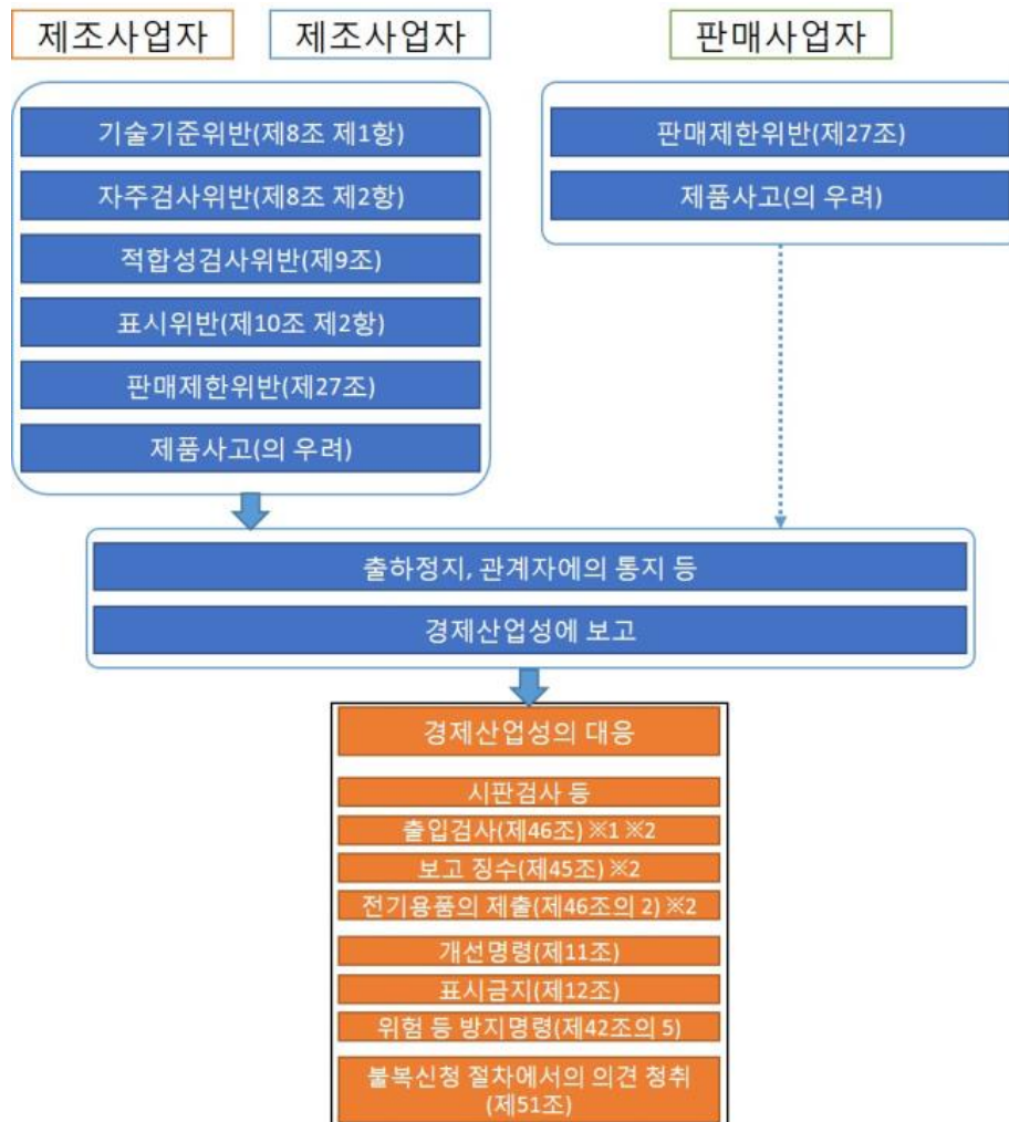
〈그림 3-14〉 전기용품안전법의 업무 절차 흐름도(제품 유통 후)
